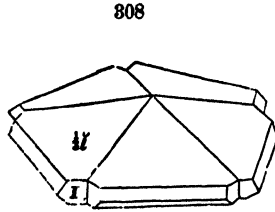
Marcasite.
